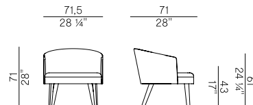
903/PL poltrona lounge \ lounge armchair
