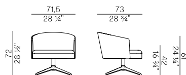
903/PLG poltrona lounge girevole \ swivel lounge armchair
