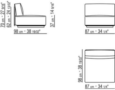
COD. 0265C0 CORNER
