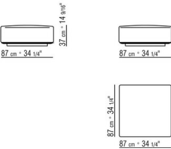
COD. 0265G0 OTTOMAN
