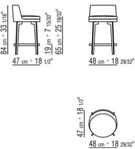
COD. 014WA7 STOOL / METAL BASE H.65
