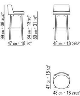
COD. 014WA4 STOOL / METAL BASE H.80
