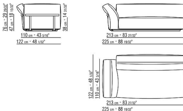
COD. 02C039 CORNER L
