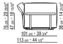
COD. 02C0F1 CORNER
