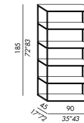
libreria - bookcase 90
