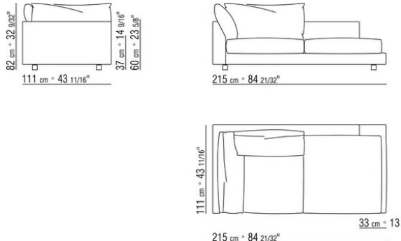
COD. 012V21 LONG CORNER L
