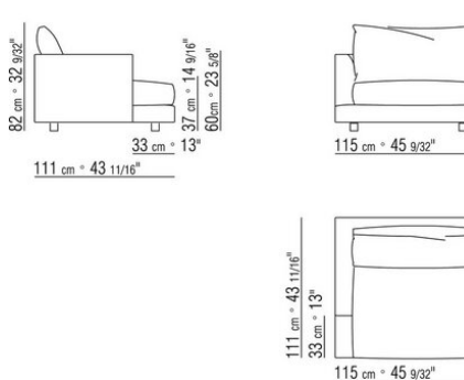
COD. 012V33 END UNIT L / DACRON
