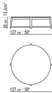
COD. 015P74 СТОЛ
