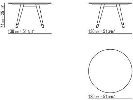
COD. 02A281 TABLE / CANALETTO BASE
