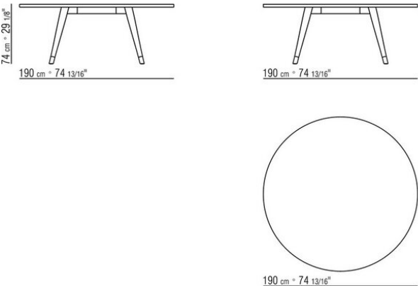
COD. 02A283 TABLE CANALETTO BASE
