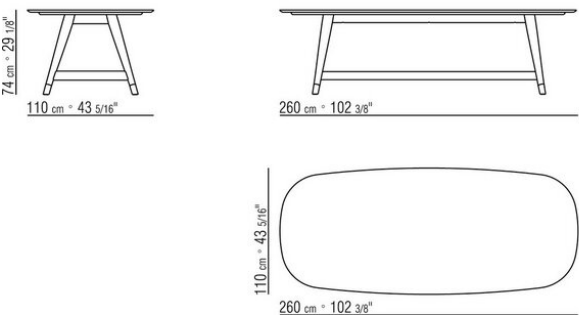
COD. 02A287 TABLE CANALETTO BASE
