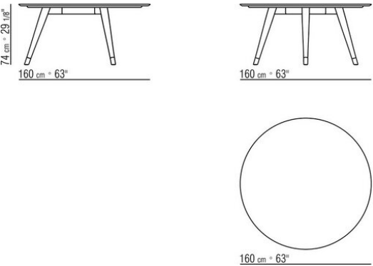
COD. 02A282 TABLE / CANALETTO BASE
