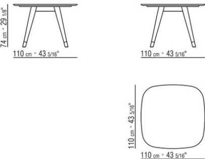
COD. 02A284 TABLE / CANALETTO BASE
