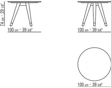
COD. 02A282 TABLE / CANALETTO BASE
