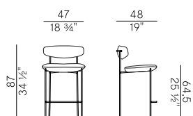
922/S sgabello basso \ counter stool
