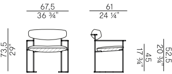
922/LMB poltrona lounge \ lounge armchair
