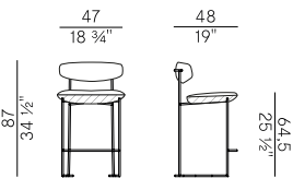
922/SMB sgabello basso \ counter stool
