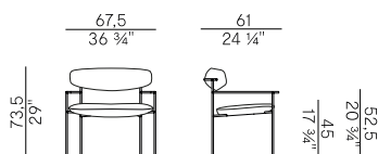
922/L poltrona lounge \ lounge armchair
