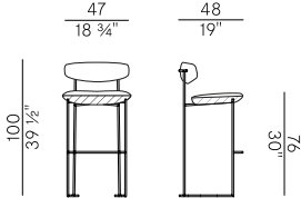
922/AMB sgabello alto \ barstool
