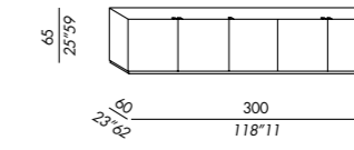
credenza - sideboard 300
