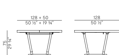
855/TC tavolo allungabile \ extendable table
