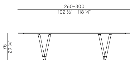
855/TR tavolo \ table
